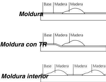
Secciones de paneles
