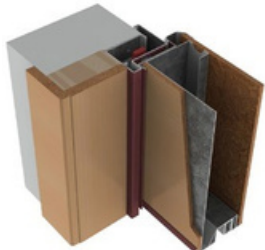
Instalación A Terminado con tapetas de MDF
