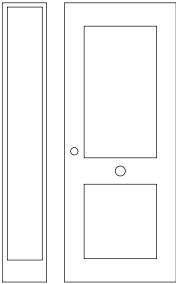
PUERTA CON UN FIJO LATERAL IZQUIERDO
